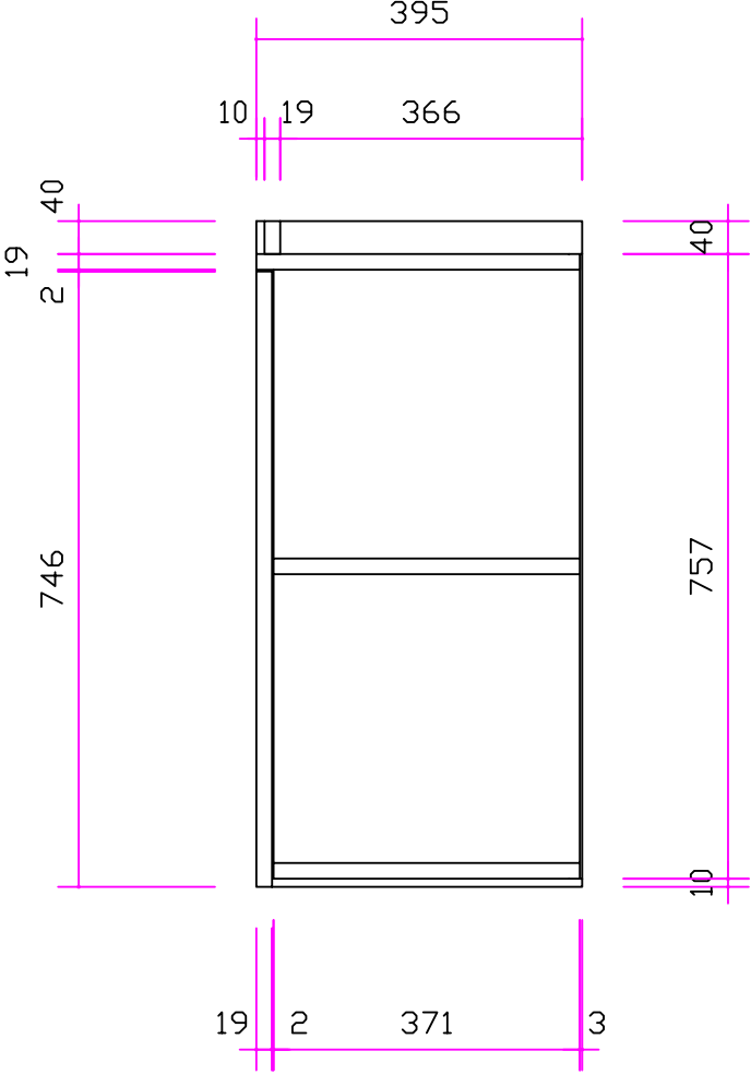
Coupe
