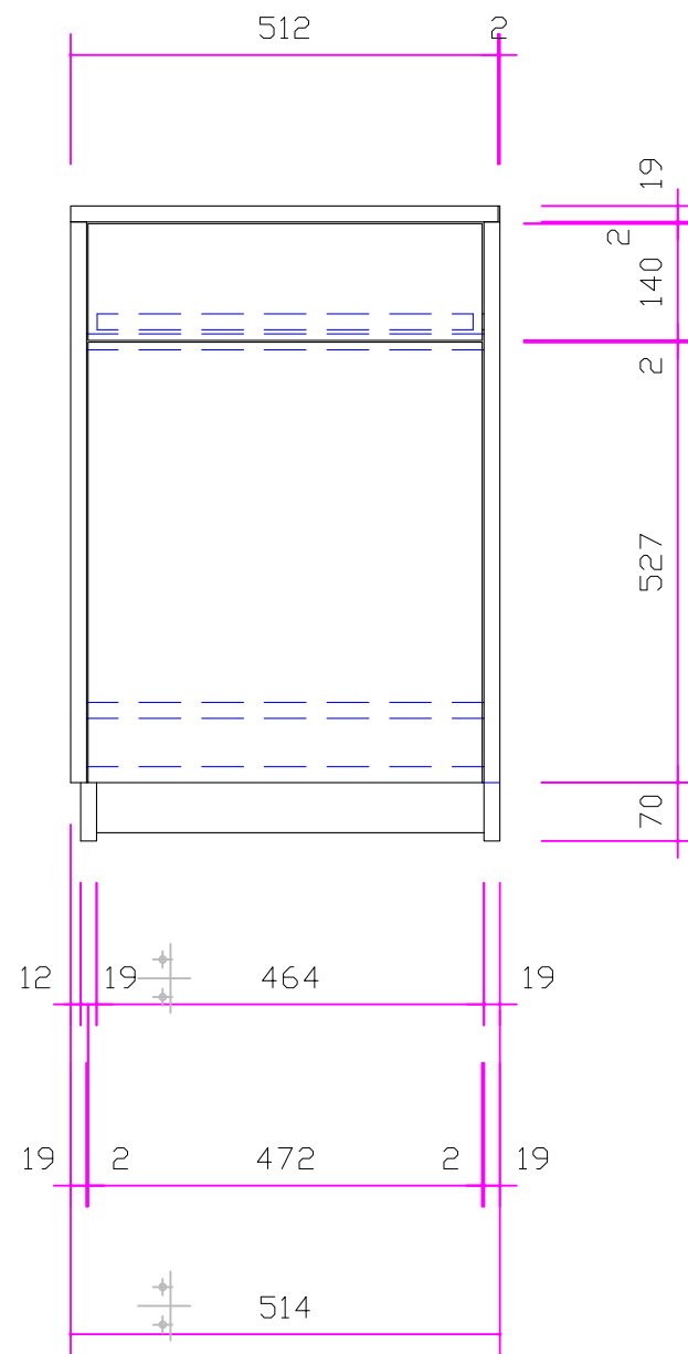
Vue avant
