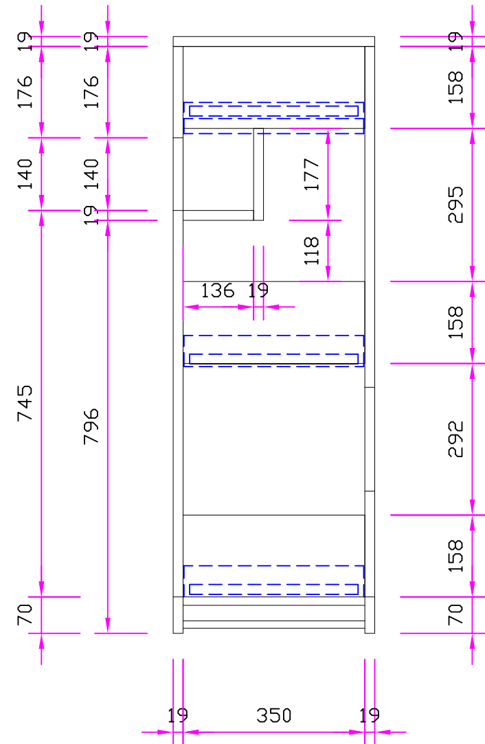
Façade arrière
