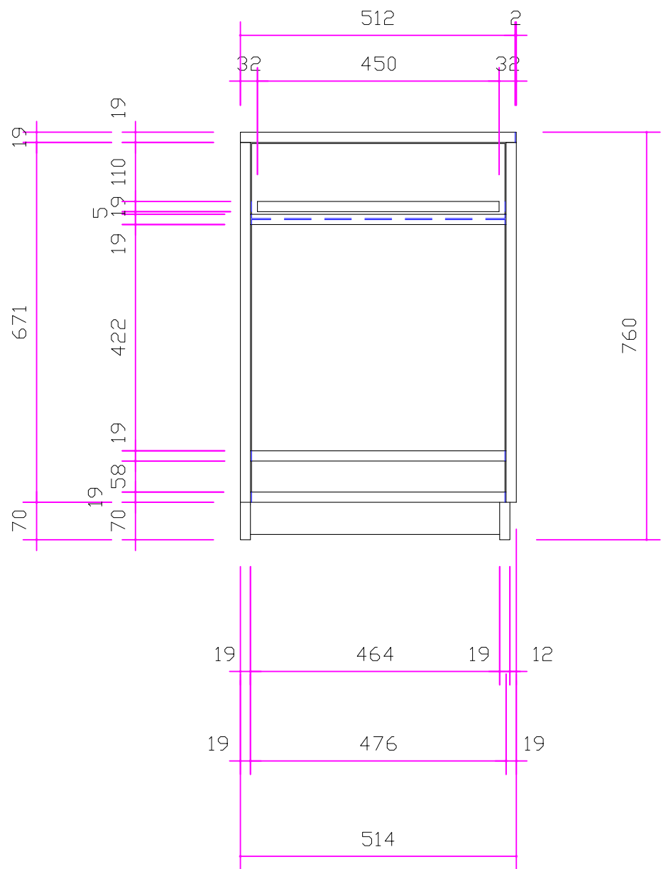
Vue arrière
