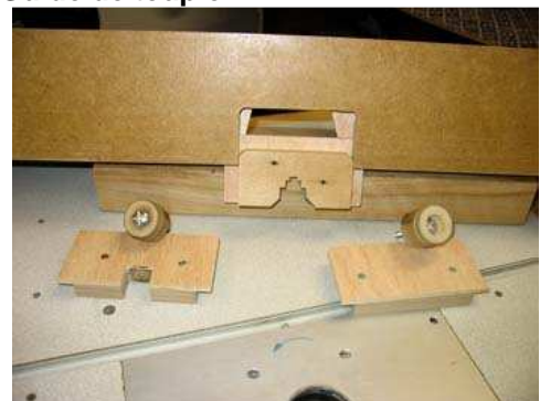
Vue Avant du guide
